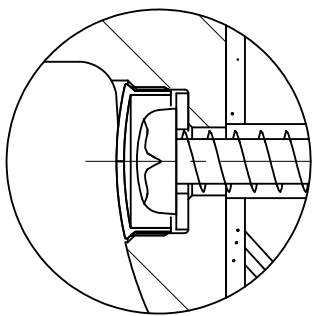
⑤ねじ隠しキャップ部詳細 (S=1/1)
