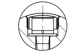
⑥ねじ隠しキャップ部詳細 (S=1/1)
